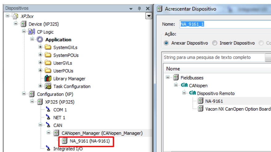
Figura 122: Adicionando um Dispositivo CANopen Escravo
