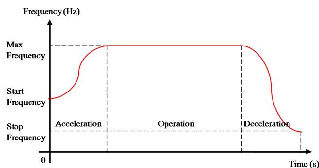
Figura 74: PTO com perfil “S”
