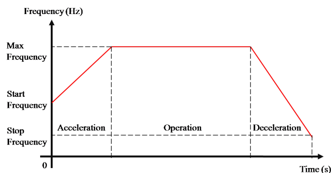
Figura 73: PTO com perfil trapezoidal
