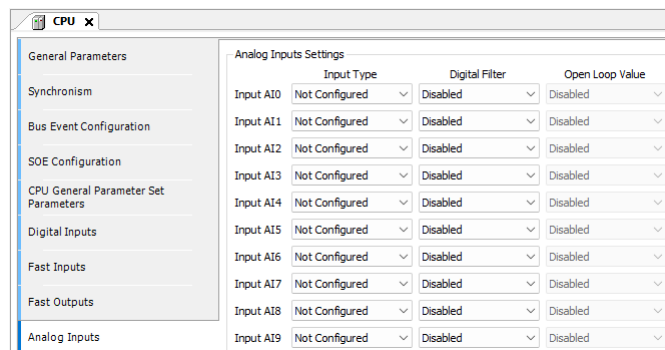
Figura 78: Parâmetros das Entradas Analógicas
