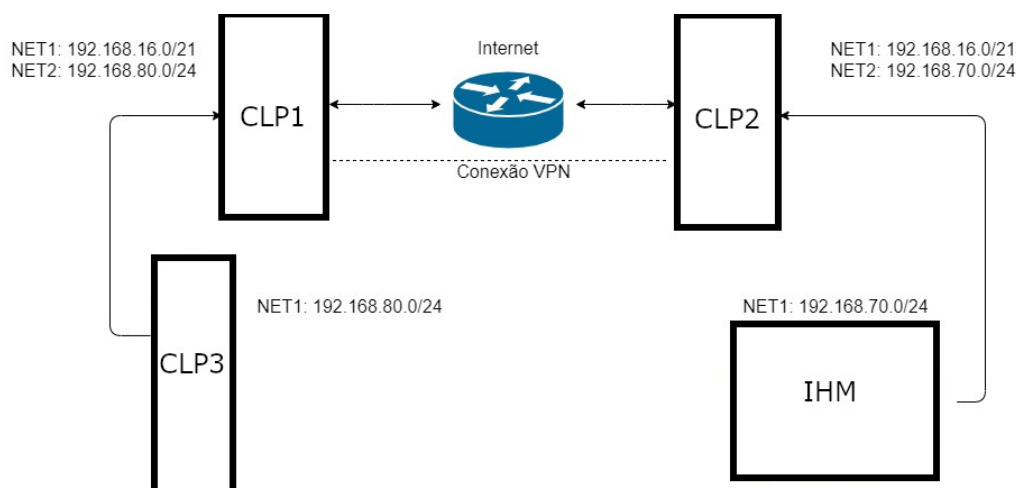
Figura 185: Exemplo de Arquitetura com Redes Privadas
