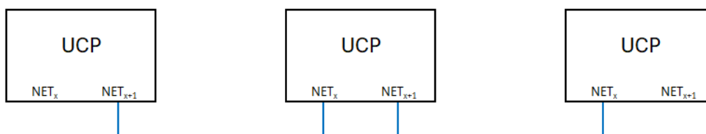
Figura 55: Exemplo de Topologia com o Modo Switch - Loop Protection Disabled
