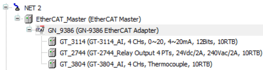
Figura 103: Exemplo de Configuração EtherCAT
