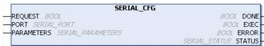
Figura 135: Bloco de Configuração da Serial
