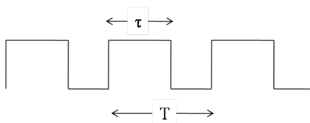
Figura 71: Forma de onda VFO/PWM
