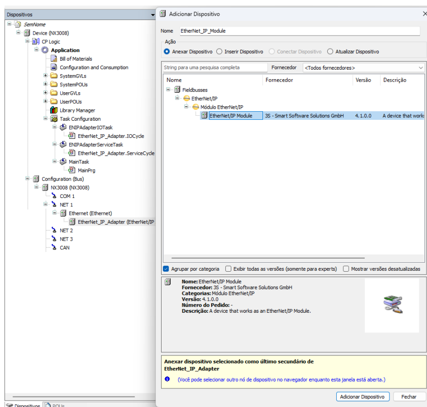
Figura 119: Adicionando um Módulo EtherNet/IP Abaixo do Adapter
