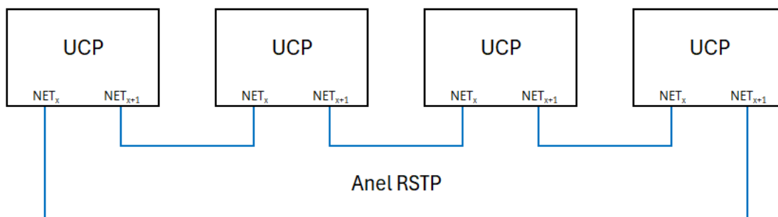
Figura 58: Exemplo de Topologia em Anel com o Modo Switch - RSTP
