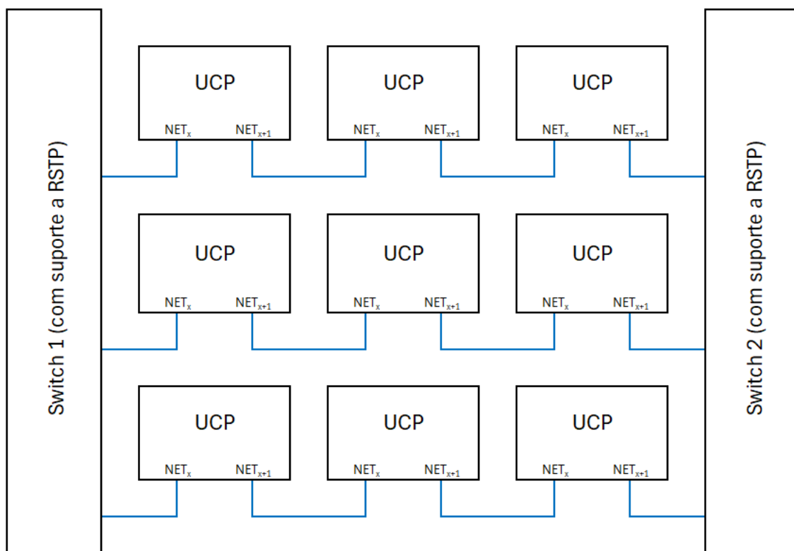
Figura 57: Exemplo de Topologia Mesh com o Modo Switch - RSTP
