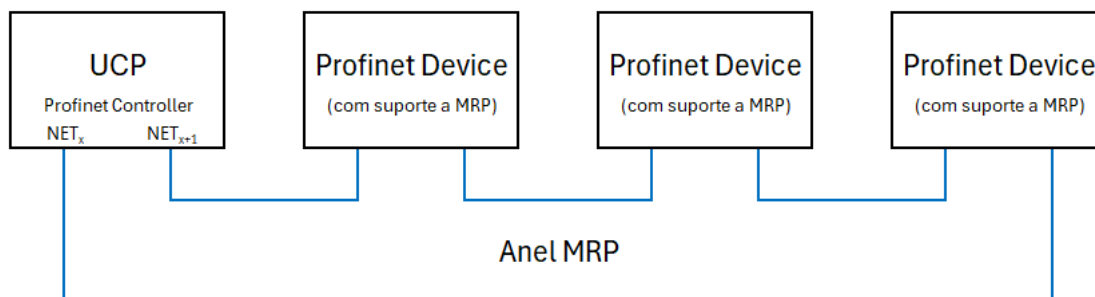
Figura 60: Exemplo de Topologia em Anel com o Modo Switch - MRP
