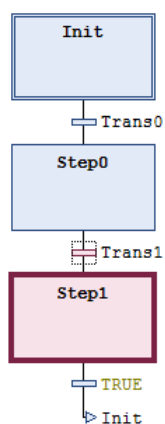
Figura 159: Transição True depois da execução do comando
