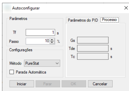
Figura 297: Autoconfigurar, Processo
