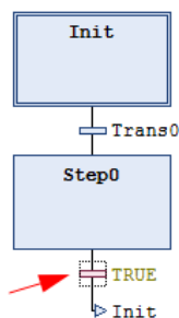
Figura 158: Transição True antes da execução do comando
