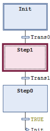
Figura 157: Depois do comando ser executado
