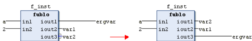
Figura 135: Alterar Conexões de Saída
