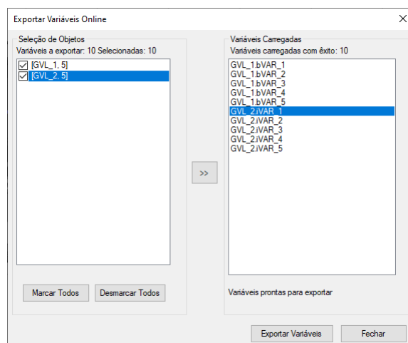
Figura 180: Variáveis a Serem Exportadas pelo Comando Exportar Variáveis Online
