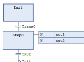
Figura 163: Associação de Ação ao Step0
