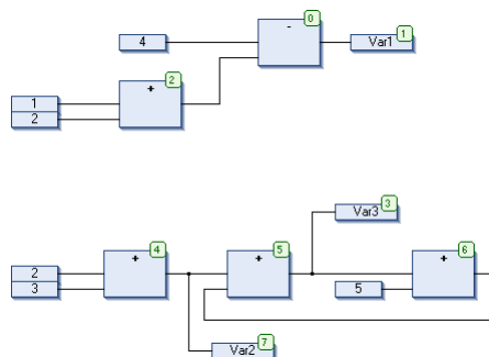
Figura 146: Ordenar por Topologia
