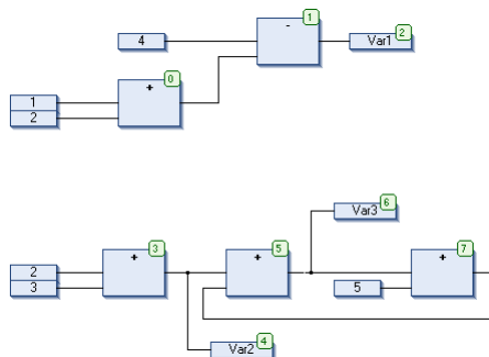
Figura 147: Processamento de Acordo com o Fluxo de Dados
