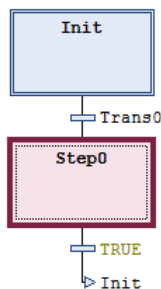
Figura 156: Antes do comando ser executado
