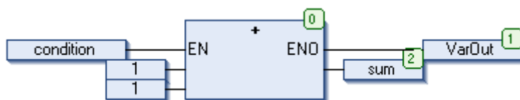
Figura 141: Caixa de Adição com EN/ENO
