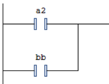
Figura 131: Contact Parallel (posição foi selecionado contato bb ) inserido em LD
