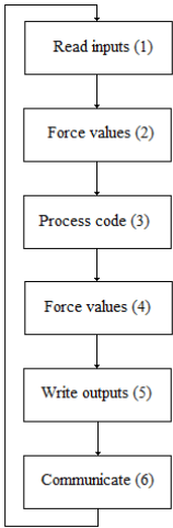
Figura 192: Sequência de Processamento em um ciclo
