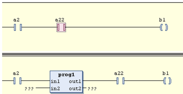
Figura 125: Inserir Bloco Funcional
