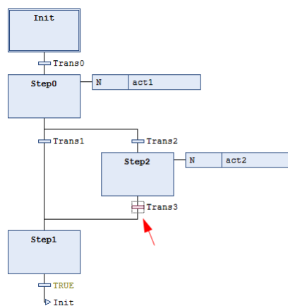
Figura 164: Comando Inserir Salto Após antes de ser executado
