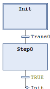
Figura 160: Etapa e Transição Inseridas
