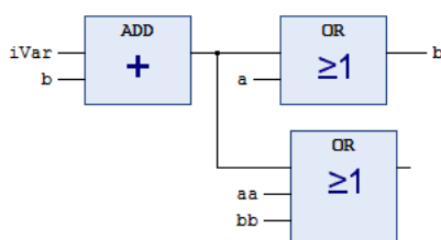
Figura 136: Marcadores de Sub-rede na Rede FBD
