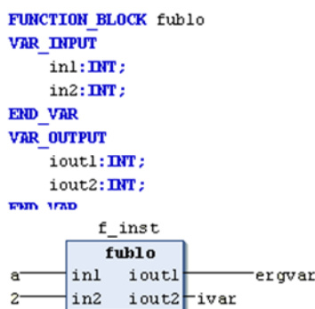
Figura 137: Versão Original do Bloco Funcional com duas saídas
