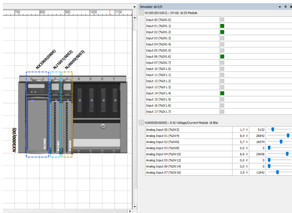
Figura 79: Simulador de E/S
