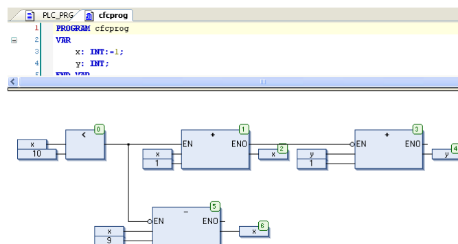
Figura 142: Uso de EN/ENO
