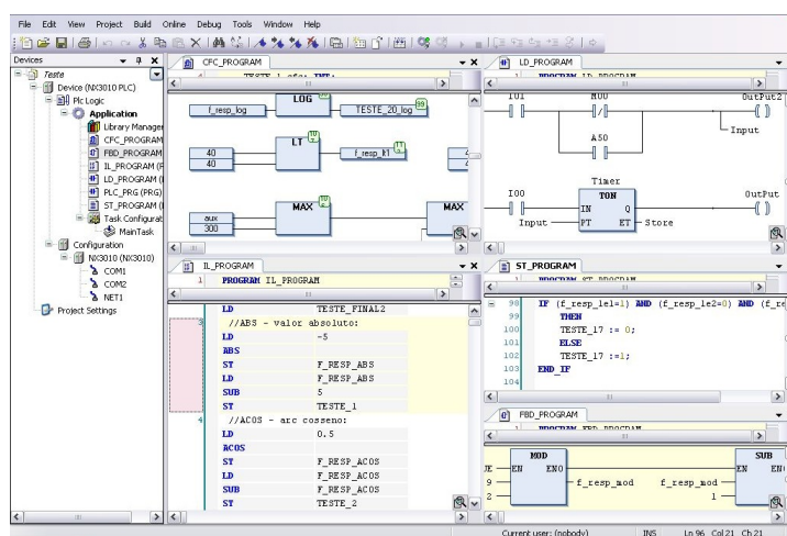
Figura 28: Linguagens de Programação IEC 61131-3
