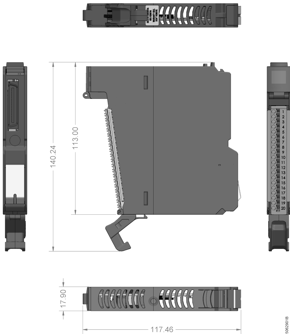
Figura 19: Módulo Nexto Jet de E/S de 18 mm
