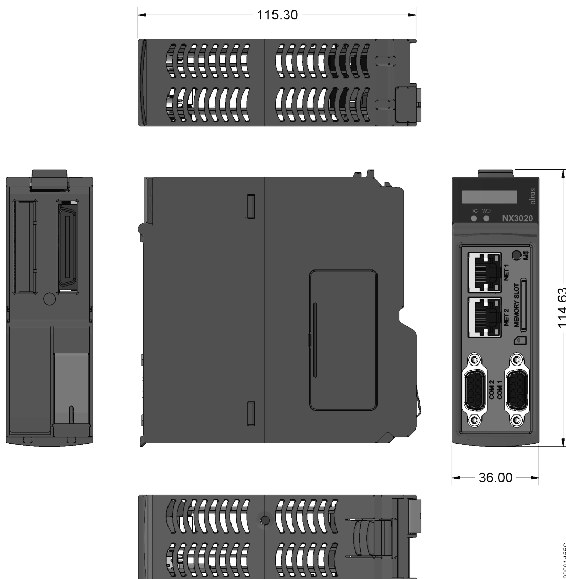
Figura 21: Módulo UCP NX3020 de 36 mm
