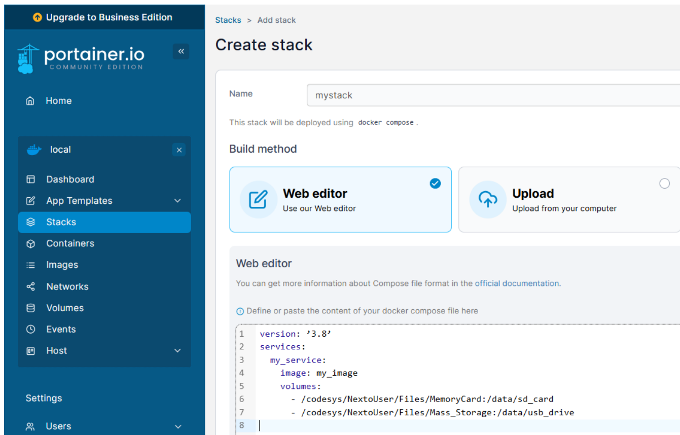
Figura 220: Exemplo de Arquivo de Stack com Memória Externa
