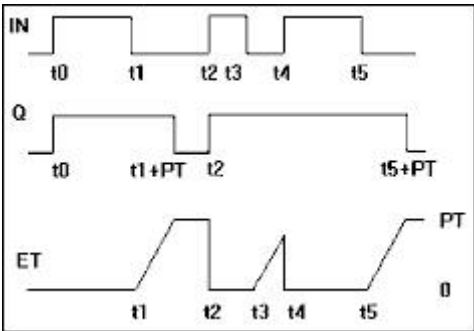
Figura 177: Comportamento Gráfico do Bloco Funcional TOF_RET
