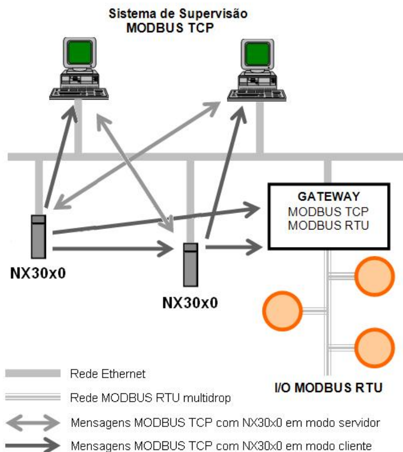
Figura 84: Rede de Comunicação MODBUS TCP
