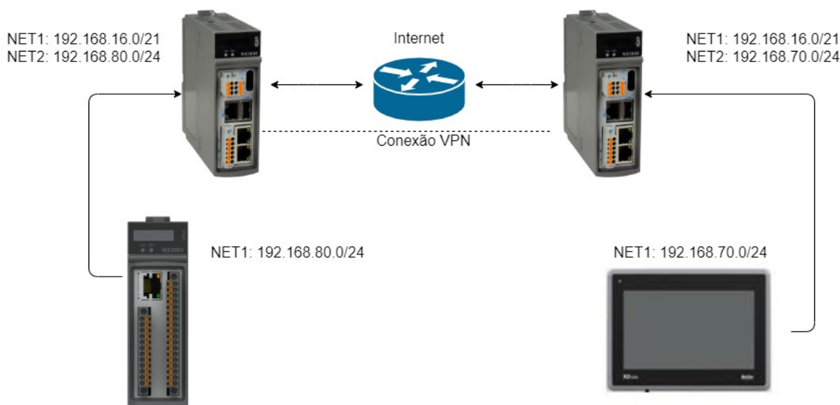
Figura 195: Exemplo de Arquitetura com Redes Privadas
