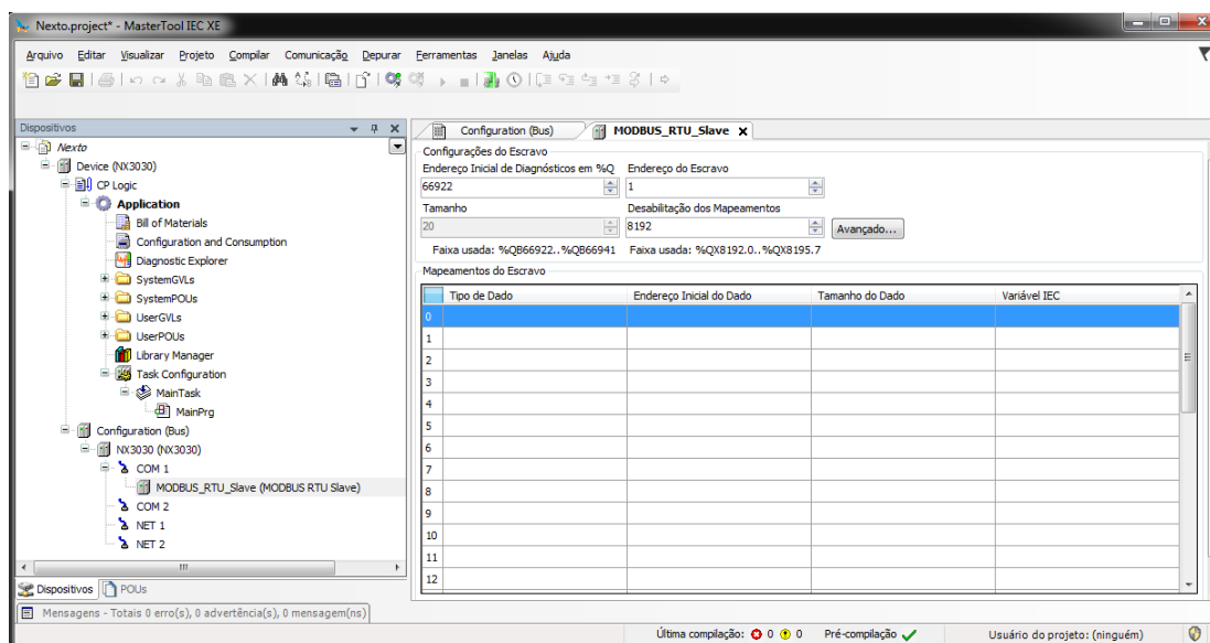
Figura 81: Tela de Configuração MODBUS RTU Escravo por Representação Direta
