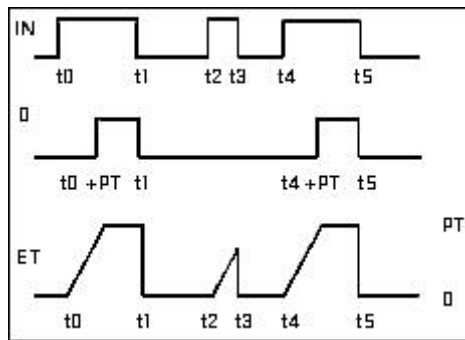
Figura 179: Comportamento Gráfico do Bloco Funcional TON_RET
