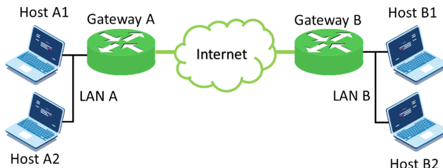
Figura 202: Exemplo de topologia Site-to-Site
