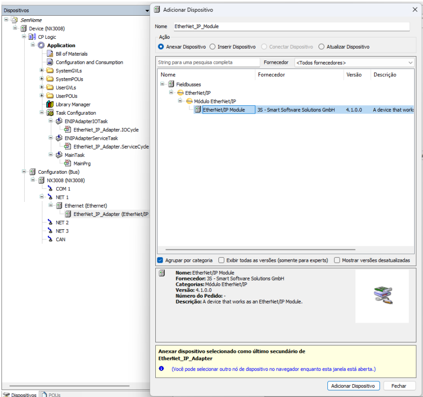
Figura 127: Adicionando um Módulo EtherNet/IP Abaixo do Adapter
