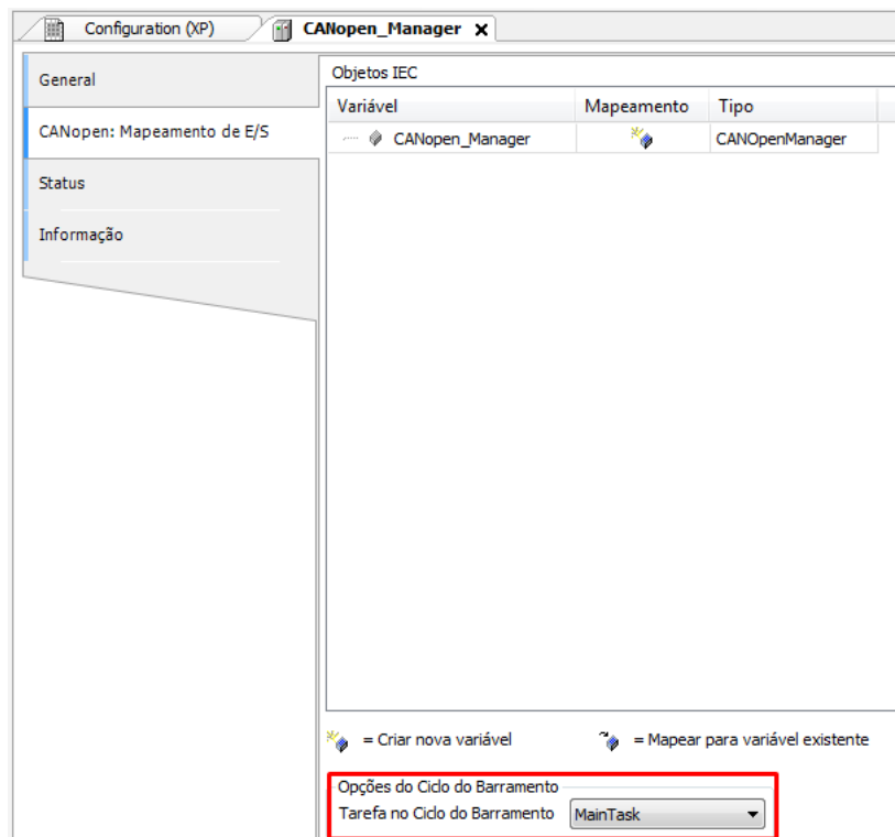
Figura 142: Configuração da tarefa cíclica do barramento CANopen
