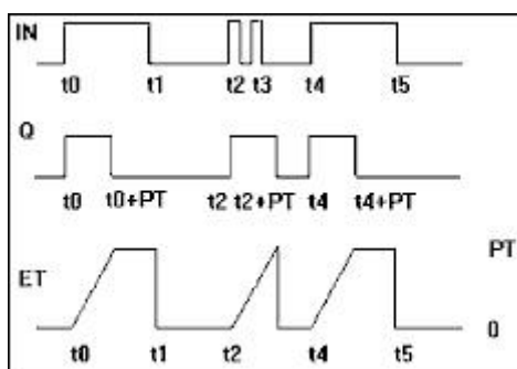
Figura 181: Comportamento Gráfico do Bloco Funcional TP_RET
