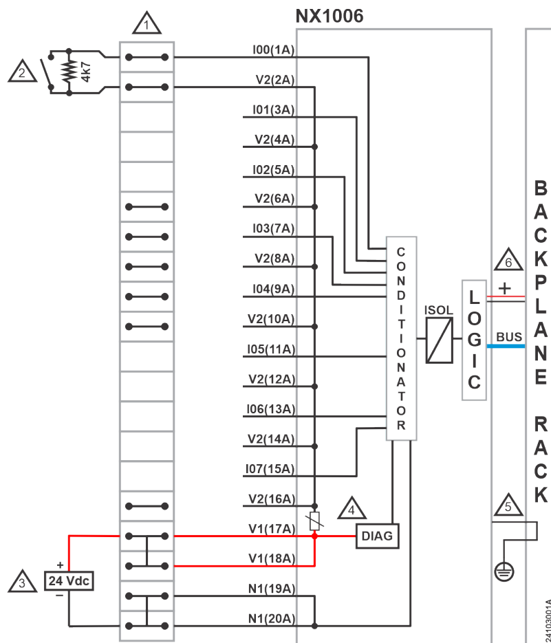
Figura 3: Diagrama Elétrico
